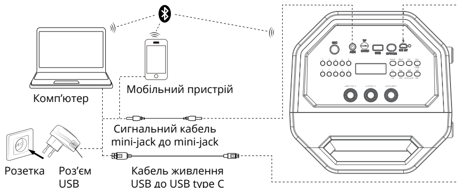
Мал. 3. Схема підключення
