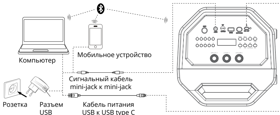
Рис. 3. Схема подключения
