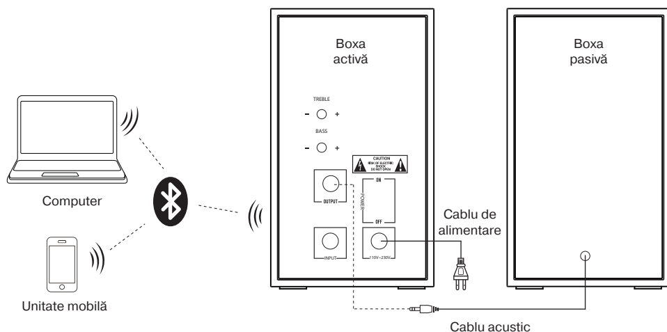
Imag. 3. Schema de conectare a surselor audio prin modulul Bluetooth
