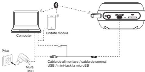
Imag. 2. Schema conectării
