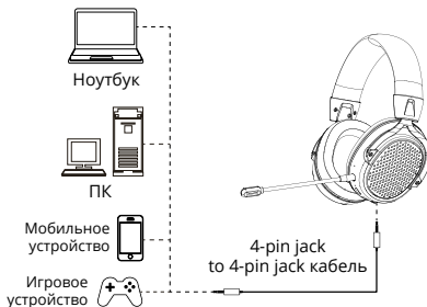
Рис. 2. Проводное подключение Line-in
