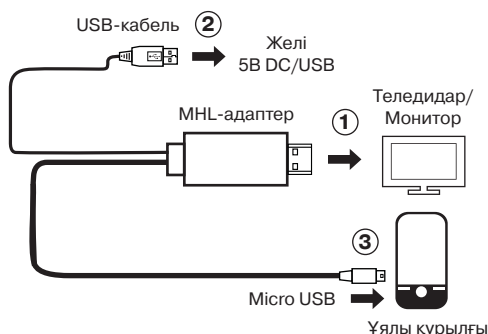
Қосылу схемасы
